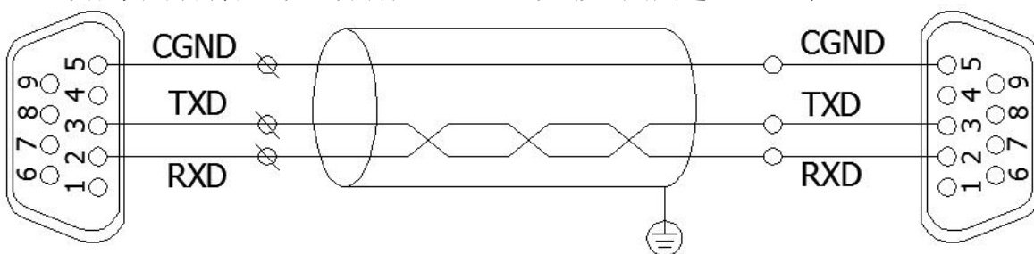
仪表侧RS232C通讯接口
